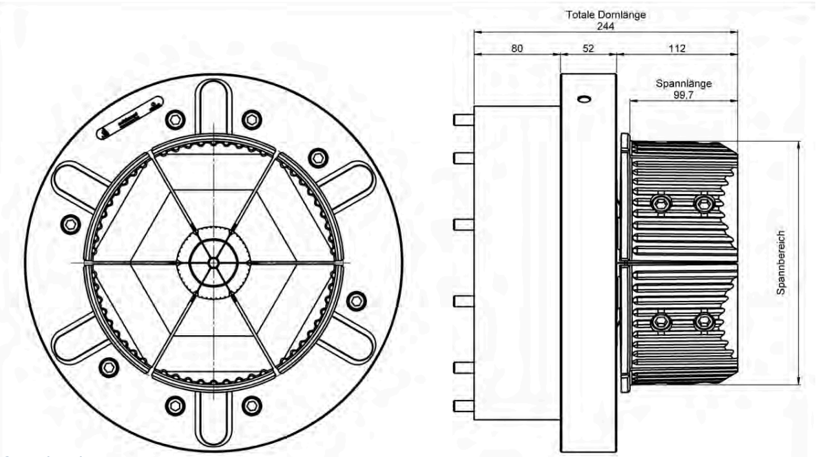
Aufsetzbacken
