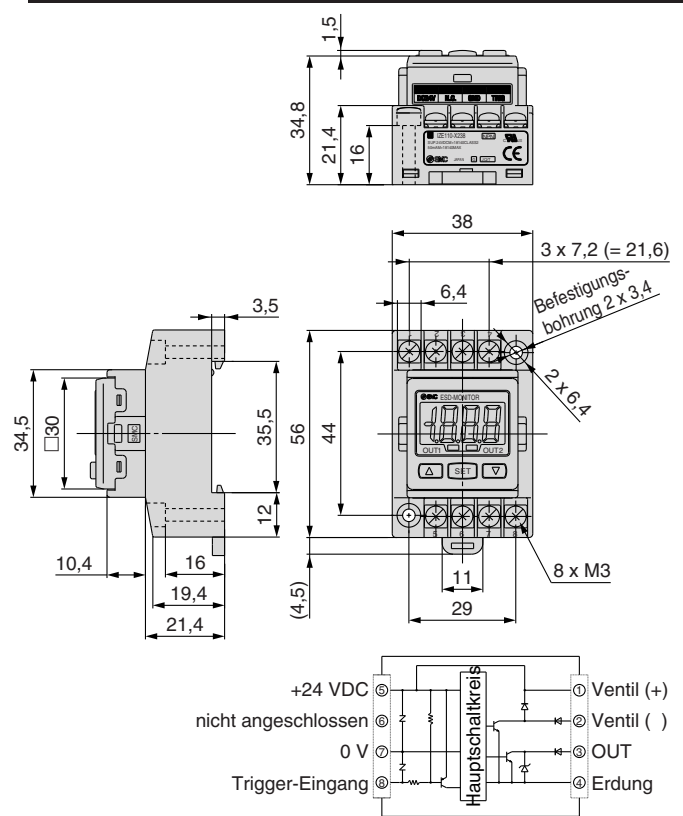
Eingangss-/Ausgangsschaltung
