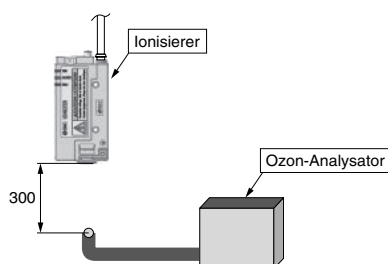
Abb. 2: Ozonkonzentration Messkreis
