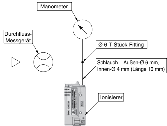
Abb. 1: Durchfluss-Kennwerte Messkreis
